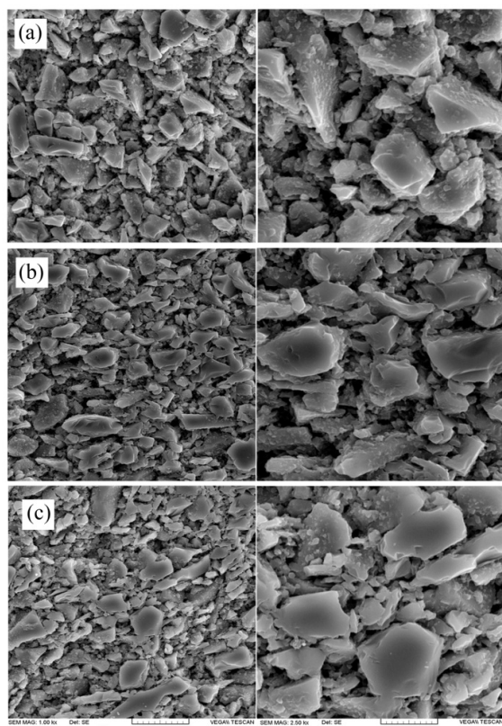
شکل ۵- تصاویر SEM نمونه‌های زینتر شده در دمای 1200^{\circ}\text{C} ۱ (a)، ۲ (b) و ۳ (c) ساعت
