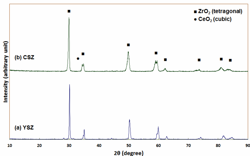
شکل ۲- آنالیز پراش پرتو ایکس از سطح YSZ و CSZ.
