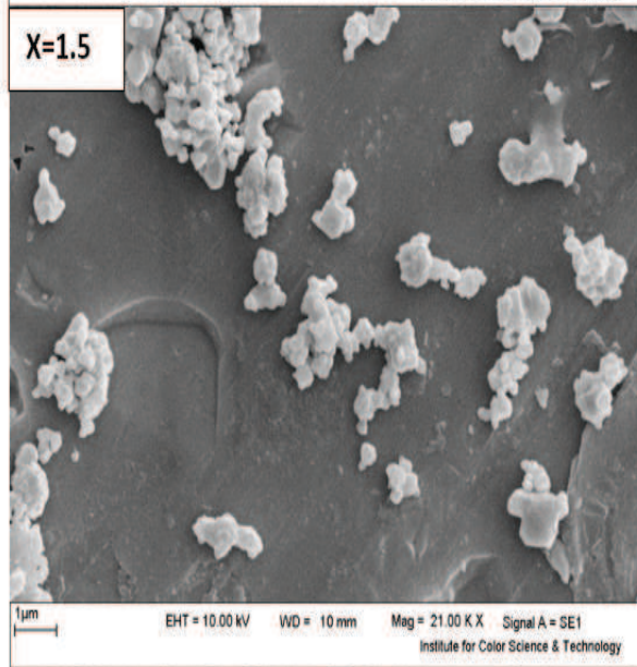
شکل ۴- ب مورفولوژی نمونه‌های سنتز شده با دوپنت منگنز پس از کلسیناسیون در دمای 1000^{\circ}\text{C} در اتمسفر معمولی
