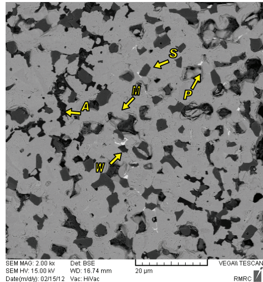
شکل ۵- تصویر SEM از نمونه \text{ZrB}_2\text{-10 wt \% nanoSiC-3 wt \% B}_4\text{C} زینتر شده در دمای 2100^\circ\text{C}
