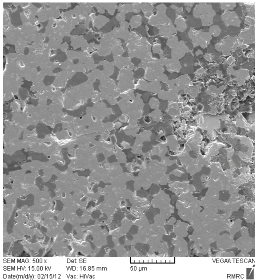
شکل ۶- تصویر SEM از مسیر حرکت ترک در نمونه \text{ZrB}_2\text{-15 wt \% SiC-3 wt \% B}_4\text{C}
