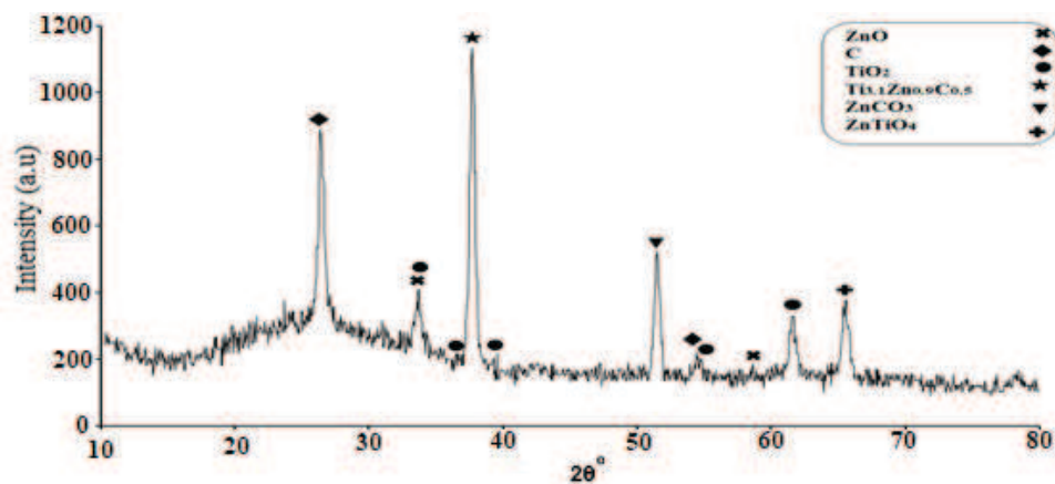
شکل ۵- نمودار پراش پرتو X (XRD) نمونه RGO-ZnO-TiO 2
