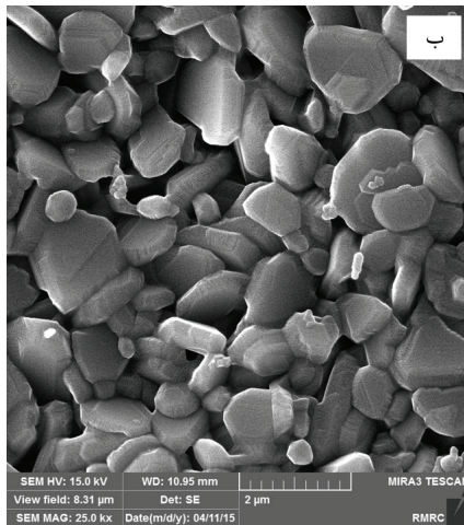
شکل ۴- تصاویر SEM اچ حرارتی نمونه‌های زینتر شده الف) خالص و ب) حاوی افزودنی‌های YSZ و اکسید نایوبیوم.
