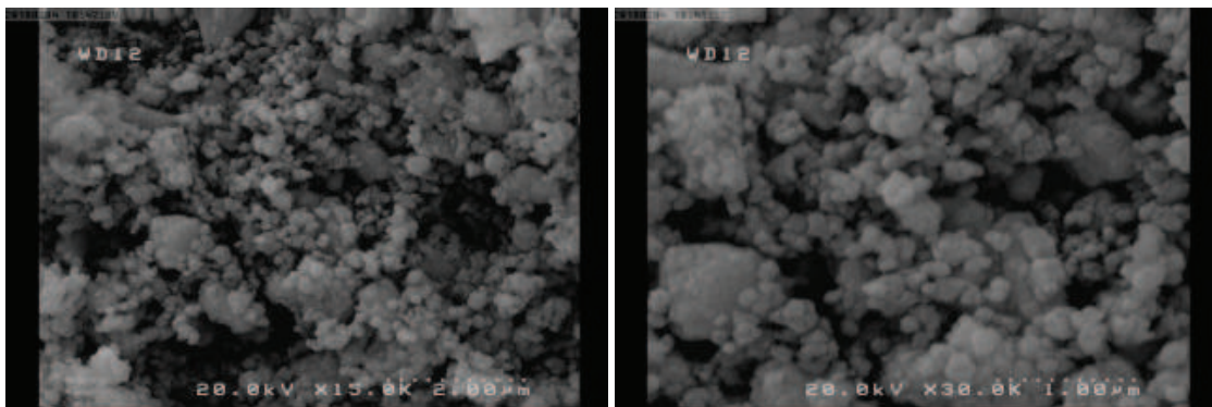
شکل ۳- تصاویر میکروسکوپی الکترونی روبشی گسیل میدانی از نانوپودر ایتریا با آلائیده به ۱ درصد نئودیمیم بزرگنمایی مختلف.
