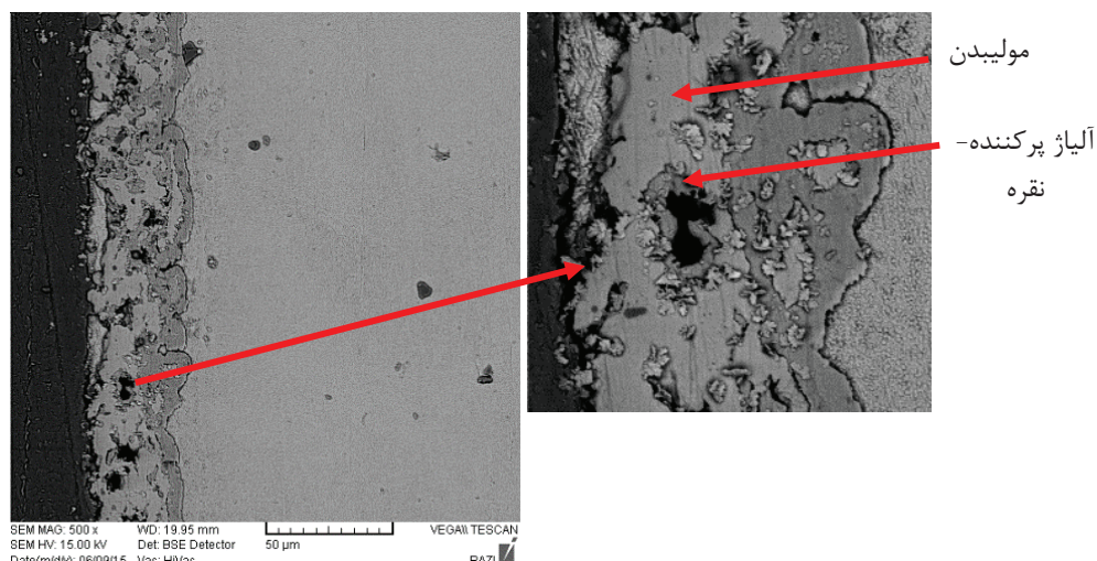
شکل ۱۰- تصویر میکروسکوپ الکترونی روبشی از فصل مشترک اتصال نمونه‌های کشش، متالایز شده تحت دمای ۱۵۰۰ درجه سانتیگراد.
