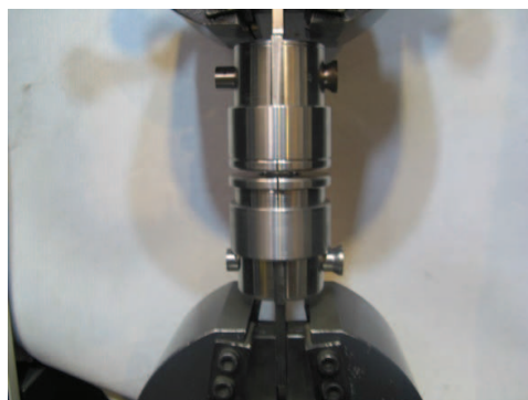
شکل ۶- آزمایش کشش برای نمونه‌های اتصال دهی شده در شکل ۴.
