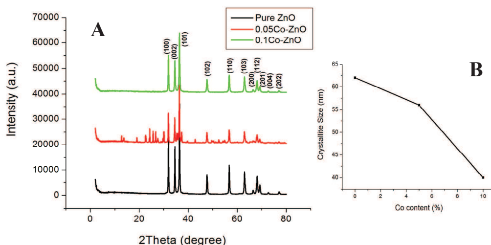
شکل ۱- الگوهای XRD مربوط به (A) ZnO خالص و به همراه ناخالصی (B) تغییرات اندازه ذره با درصد ناخالصی Co
