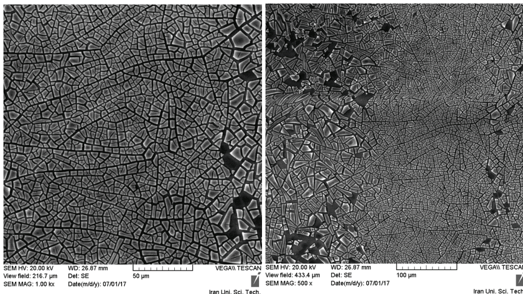
شکل ۹- تصاویر SEM پوشش تیتانیای دوپ شده با فلئور در دو بزرگنمایی ۲۰۰ و ۵۰۰ برابر
