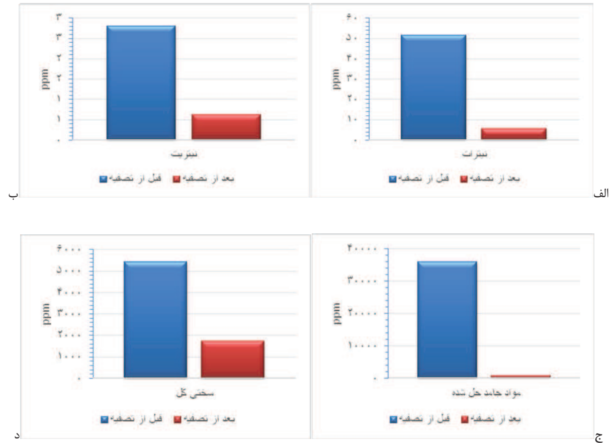
شکل ۷- (الف): میزان تغییرات نیترات با استفاده از فیلتر نمونه شماره ۷ با قطر ۲۰ میلی‌متر (ب): میزان تغییرات نیتريت با استفاده از فیلتر نمونه شماره ۷ با قطر ۲۰ میلی‌متر (ج): میزان تغییرات مواد جامد حل شده با استفاده از فیلتر نمونه شماره ۷ با قطر ۲۰ میلی‌متر (د): میزان تغییرات سختی کل با استفاده از فیلتر نمونه شماره ۷ با قطر ۲۰ میلی‌متر
