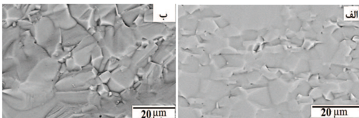
شکل ۲- تصاویر SEM از سطح شکست قطعه یگ شفاف، الف) قبل از آنیل ب) بعد از فرآیند آنیل
