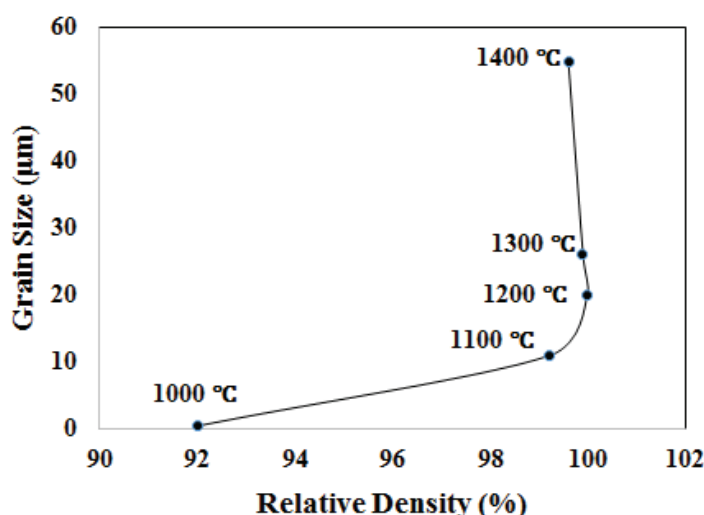
شکل ۲- اندازه دانه‌های نمونه‌های منیزیای زینتر شده در مقابل دانسیته نسبی آن‌ها در دماهای مختلف در زمان ۲۰ دقیقه با فشار اعمالی ۸۰ مگاپاسکال در طی زینتر قوس پلاسما
