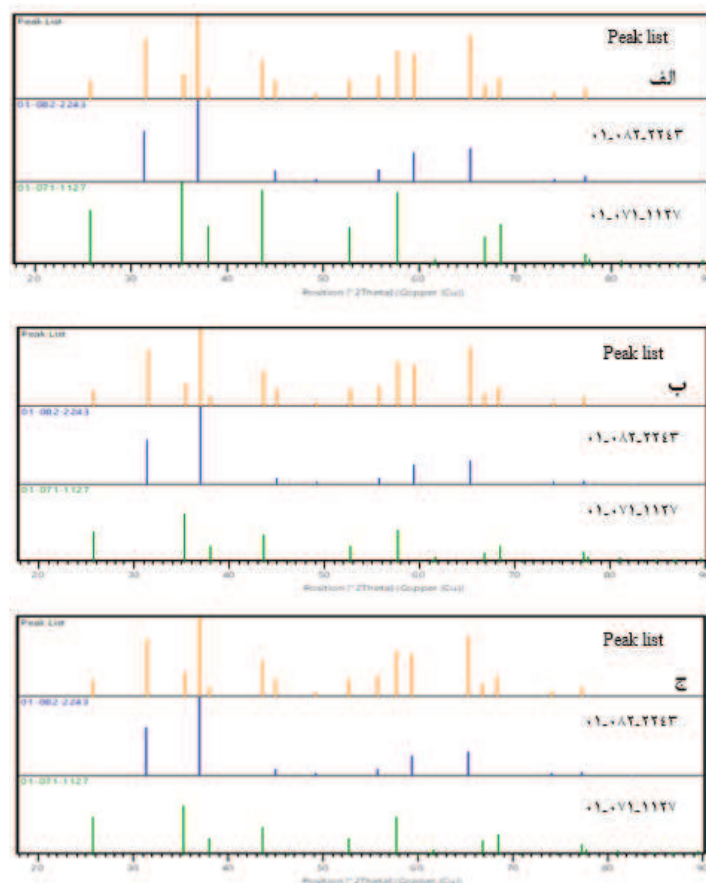
شکل ۲- تصاویر به دست آمده از آنالیزهای XRD برای مقایسه قله‌های مرجع و نمونه‌های الف) A_1 ب) A_2 ج) A_3
