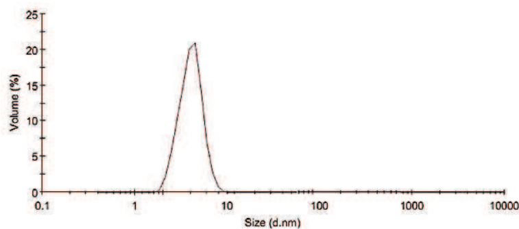
شکل ۳- منحنی توزیع اندازه ذرات پیش سازنده در داخل سل در pH=۵
