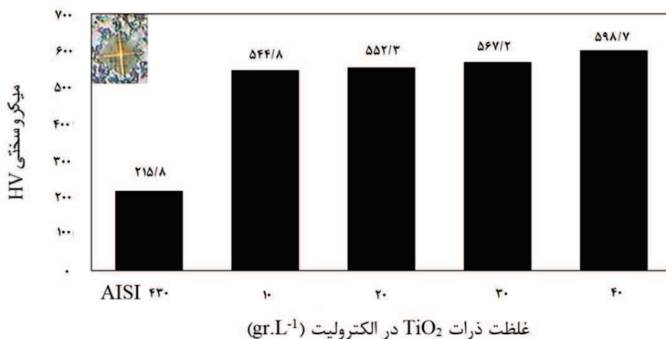
شکل ۶- تاثیر غلظت ذرات TiO 2 در الکترولیت بر میکروسختی پوشش کامپوزیتی
