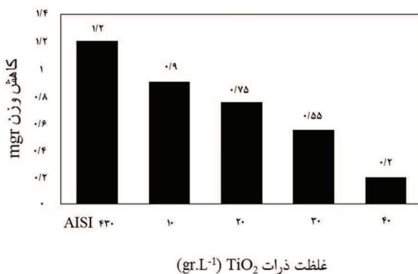
شکل ۷- تأثیر مقدار کاهش وزن نمونه ها را با تغییر غلظت ذرات \text{TiO}_2 در الکترولیت، تحت دانسیته جریان 15 \text{ mA.cm}^{-2} و \text{pH}=3/5 .
