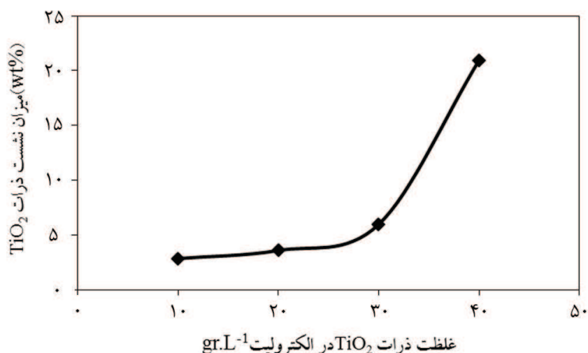
شکل ۲- تأثیر غلظت حمام بر نشست ذرات \text{TiO}_2 در \text{pH}=3/5 و جریان 15 \text{ mA.cm}^{-2}
