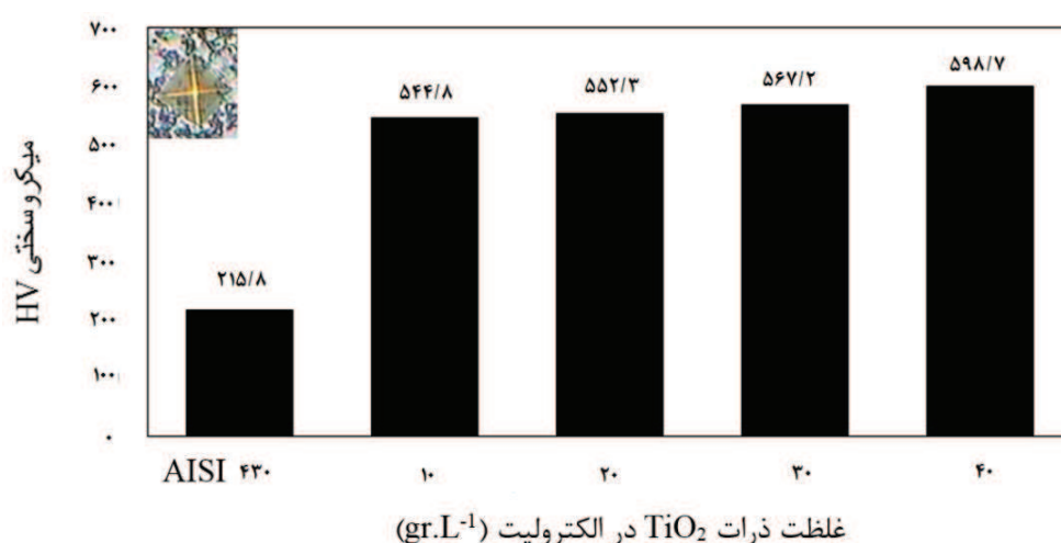
شکل ۶- تاثیر غلظت ذرات \text{TiO}_2 در الکترولیت بر میکروسختی پوشش کامپوزیتی
