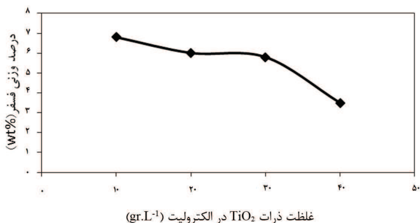
شکل ۳- تاثیر غلظت \text{TiO}_2 در الکترولیت بر میزان نشست فسفر در پوشش
