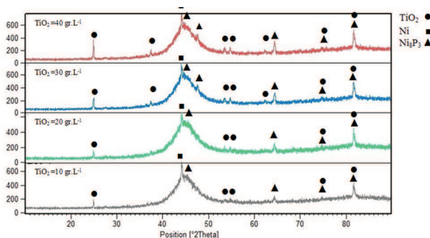
شکل ۴- نتایج XRD در غلظت‌های مختلف ذرات \text{TiO}_2 در الکترولیت
