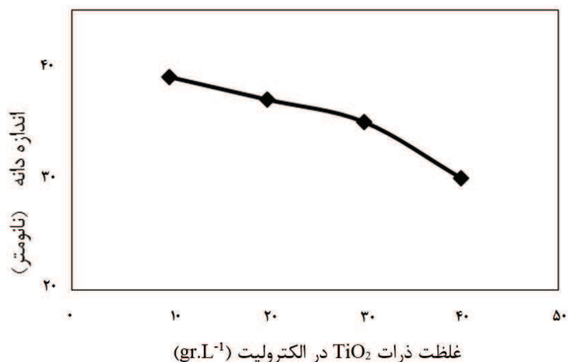
شکل ۵- تاثیر غلظت ذرات \text{TiO}_2 در الکترولیت بر اندازه دانه پوشش کامپوزیتی
