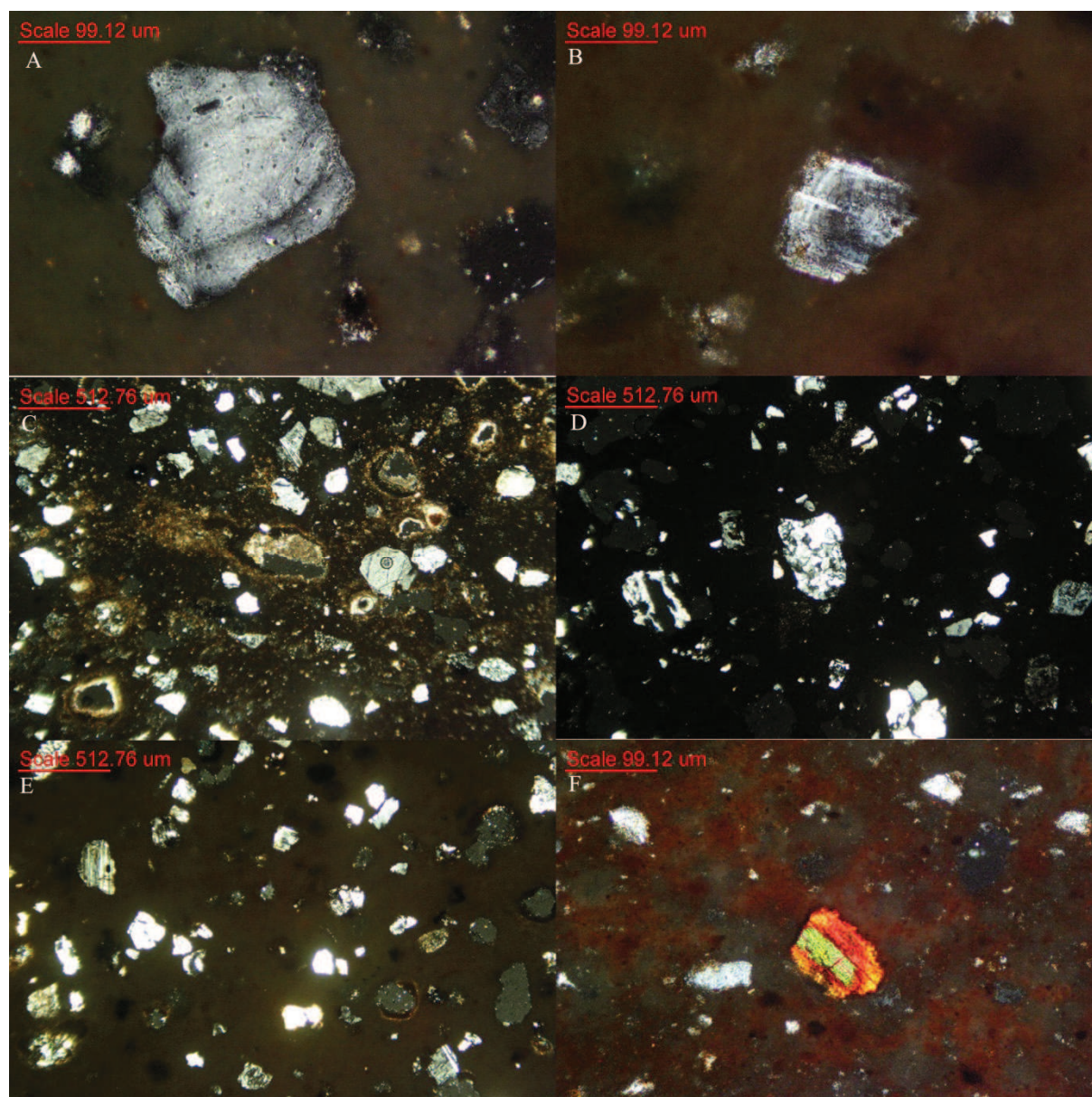
شکل ۴- (A) پدیده میرمکیتی شدن فلدسپات‌ها (2Pol-X40). (B) فلدسپات با خاصیت پدیده زون افکت (2Pol-X20). (C) پراکندگی کانی‌ها در نور XPL (2Pol-X40). (D) کوارتز با منشا متامورف (2Pol-X10). (E) پراکندگی دانه‌های پرکننده کوارتز، کربنات‌ها و پلاژیوکلازها در بافت زمینه، مربوط به نمونه ۲۳۲، (2Pol-X40). (F) کانی مسکوویت در حال از دست دادن خواص نوری در بافت زمینه رسی قرمز رنگ، مربوط به نمونه ۱۰۸، (2Pol-X20).
