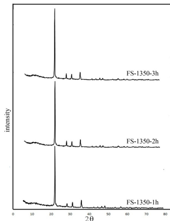
شکل ۴- الگوی پراش اشعه ایکس نمونه‌های زینتر شده در دمای 1350^{\circ}\text{C}
