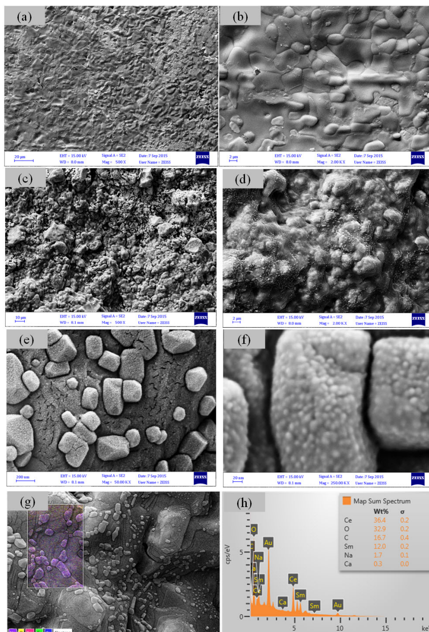
شکل ۴- تصاویر FE-SEM از نمونه‌های زیرتر شده (a) و (b) CSDC 5 و (c)، (d)، (e) و (f) کامپوزیت CSDC 5 – LN در بزرگنمایی‌های مختلف، (g) و (h) آنالیز EDX از سطح نمونه کامپوزیت.
