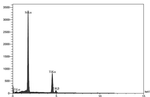
شکل ۱۰- آنالیز طیف‌سنجی پراش انرژی پرتو ایکس نقطه C مشخص شده در شکل (۷، ج).
