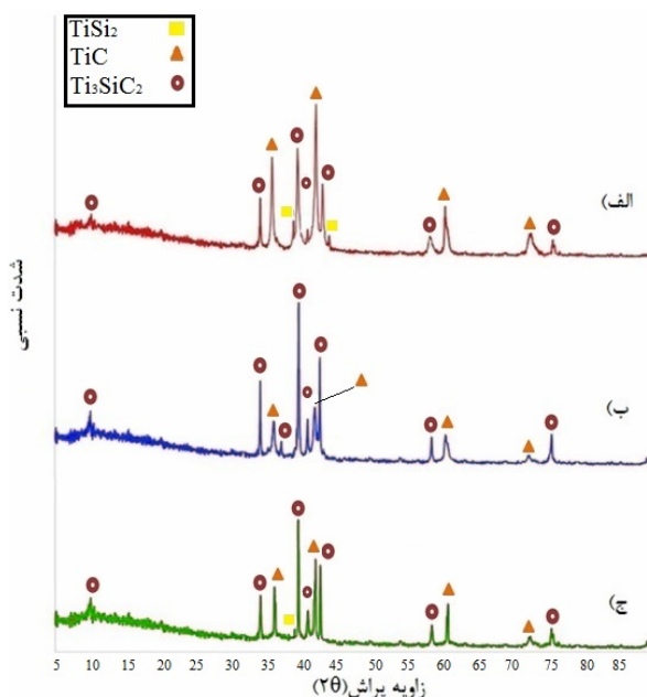
شکل ۵- الگوهای XRD برای نمونه‌های عملیات حرارتی شده در دماهای
