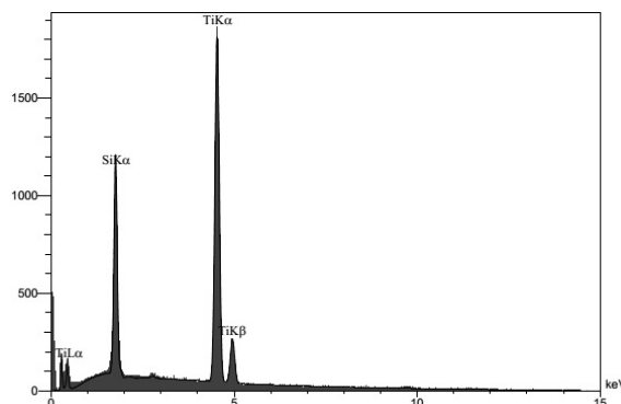
شکل ۸- آنالیز EDS نقطه A مشخص شده در شکل (۷، ج).
