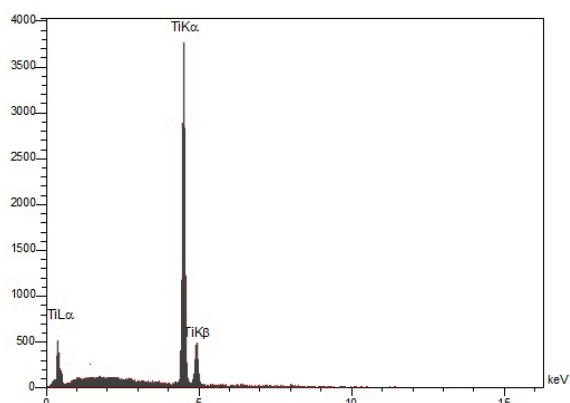
شکل ۹- آنالیز طیف‌سنجی پراش انرژی پرتو ایکس نقطه A مشخص شده در شکل (۷، ج).
