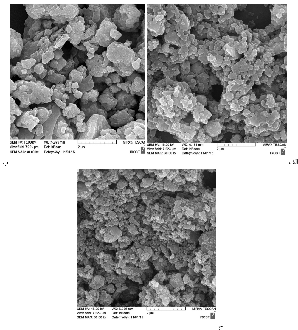
شکل ۲- تصاویر میکروسکوپ الکترونی روبشی از نمونه‌های آسیاکاری شده در مدت زمان‌های مختلف: (الف) ۳۰ ساعت، (ب) ۴۰ ساعت و (ج) ۵۰ ساعت.
