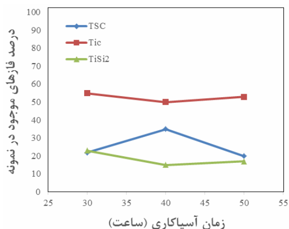
شکل ۴- درصد فازهای موجود در نمونه های عملیات حرارتی شده در دمای ۱۱۰۰ °C به مدت یک ساعت برحسب تغییرات زمان آسیاکاری بر اساس روش ریتولد.
