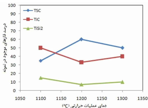
شکل ۶- درصد فازهای موجود در نمونه‌های عملیات حرارتی شده برحسب تغییرات دمای عملیات حرارتی بر اساس روش ریتولد.
