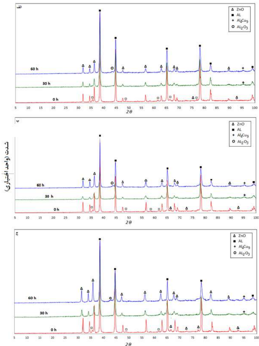
شکل ۱- الگوی پراش اشعه ایکس در زمان‌های مختلف آسیاکاری
