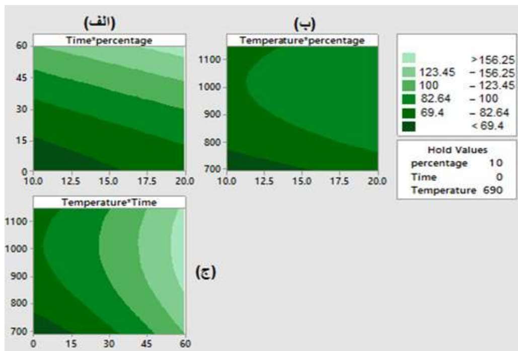
شکل ۴- نمودار هم تراز سختی بر حسب پارامترهای دمای زینتر، زمان آسیاکاری و درصد اکسید روی در شرایط:
