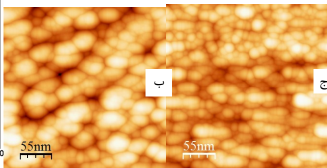
شکل ۱- الف) تغییرات فراوانی نانوذرات پوشش‌های لایه‌نشانی شده کربن-نیکل در زمان‌های ۵۰، ۹۰، ۱۸۰ و ۶۰۰ ثانیه بر حسب توپوگرافی سطح و تصاویر AFM پوشش‌های لایه‌نشانی شده کربن-نیکل در ب) ۱۸۰ ثانیه و ج) ۶۰۰ ثانیه.
