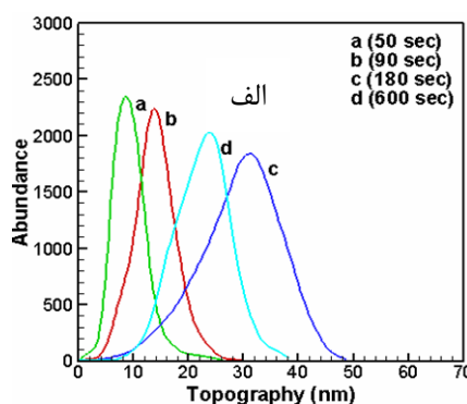
شکل ۱- الف) تغییرات فراوانی نانوذرات پوشش‌های لایه‌نشانی شده کربن-نیکل در زمان‌های ۵۰، ۹۰، ۱۸۰ و ۶۰۰ ثانیه بر حسب توپوگرافی سطح و تصاویر AFM پوشش‌های لایه‌نشانی شده کربن-نیکل در ب) ۱۸۰ ثانیه و ج) ۶۰۰ ثانیه.
