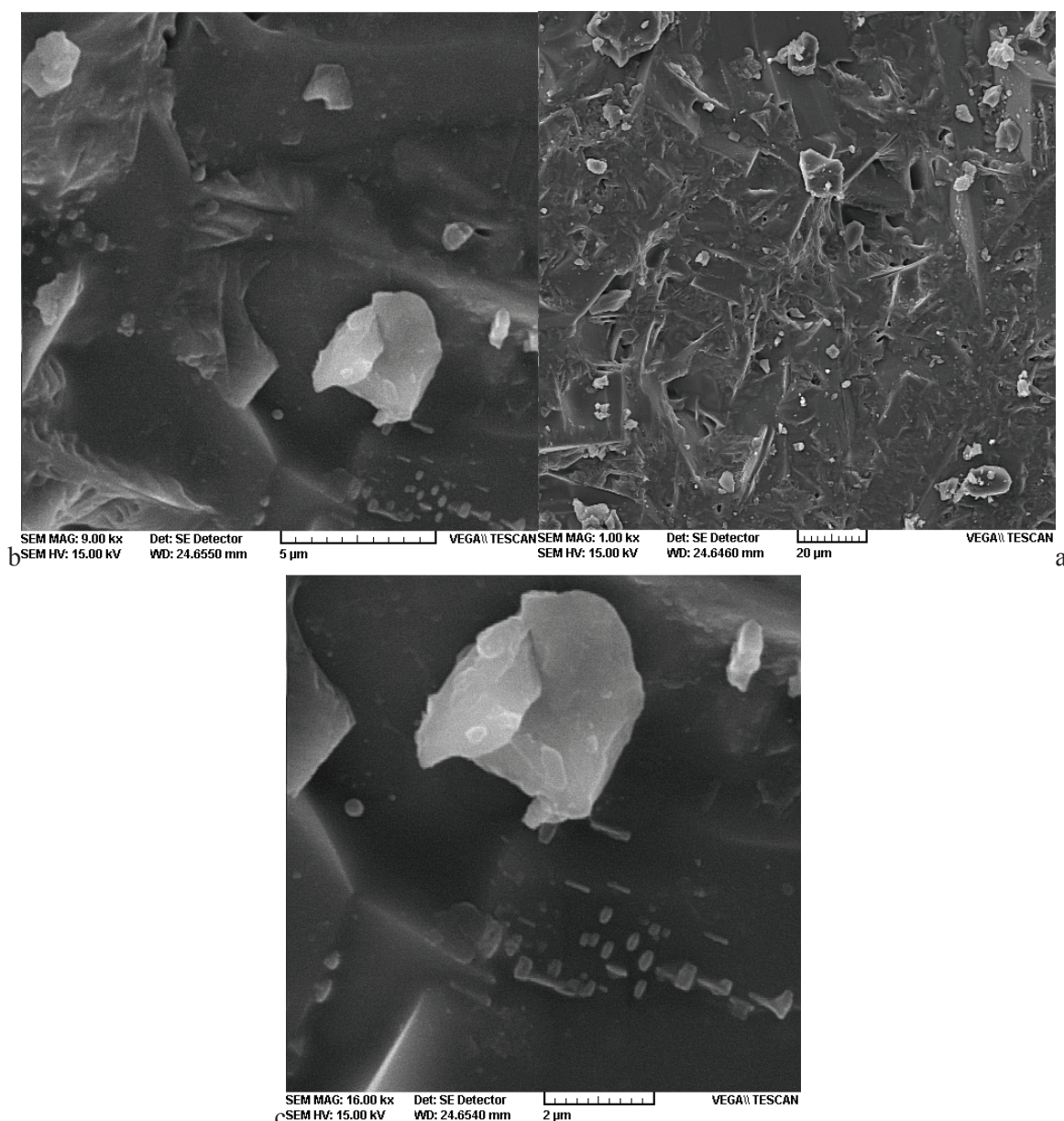
شکل ۱۴- تصاویر میکروسکوپ الکترونی روبشی نمونه V_{13} .
