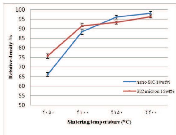
شکل ۴- تغییرات دانسیته نسبی با تغییرات دما
