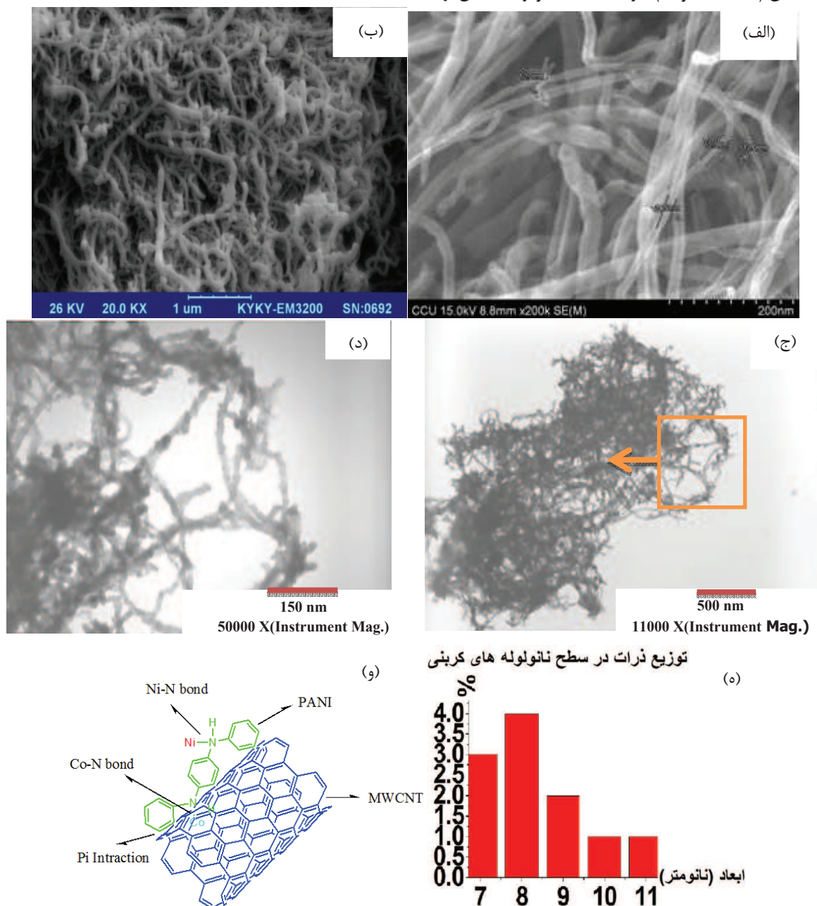
شکل ۲- الف- تصویر SEM از نانولوله‌های کربنی ب- تصویر SEM از نانوساختار PANI- CNT ج- د- تصویر TEM از نانوساختار PANI- CNT (Ni, Co) oxide ه- منحنی ستونی توزیع اندازه نانوذرات رسوب داده شده بر سطح PANI- CNT و- شماتیک نانوکامپوزیت نهایی
