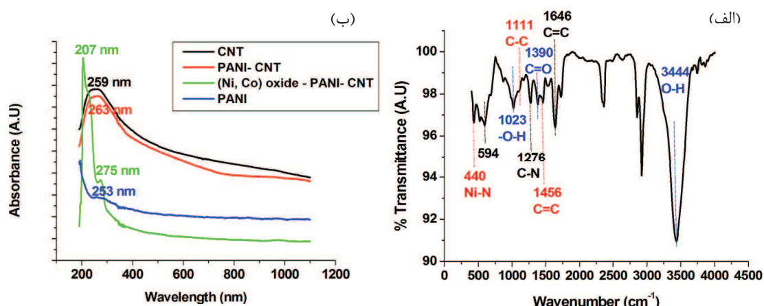
شکل ۱- (الف)- طیف FTIR حاصل از نانوکامپوزیت (Ni, Co) oxide - PANI- CNT (ب)- طیف مرئی - فرابنفش حاصل از CNT, PANI, PANI- CNT و نانوکامپوزیت (Ni, Co) oxide - PANI- CNT
