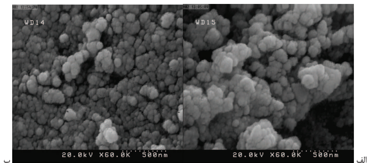
شکل ۴- تصاویر ریز ساختاری نانوذرات (الف) \text{MnFe}_2\text{O}_4 و (ب) \text{Mn}_{0.7}\text{Co}_{0.3}\text{Fe}_2\text{O}_4
