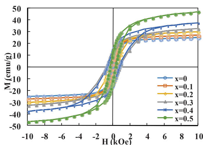
شکل ۵- حلقه هیستریزاس پودرهای هم‌رسوبی شده \text{Mn}_{1-x}\text{Co}_x\text{Fe}_2\text{O}_4
