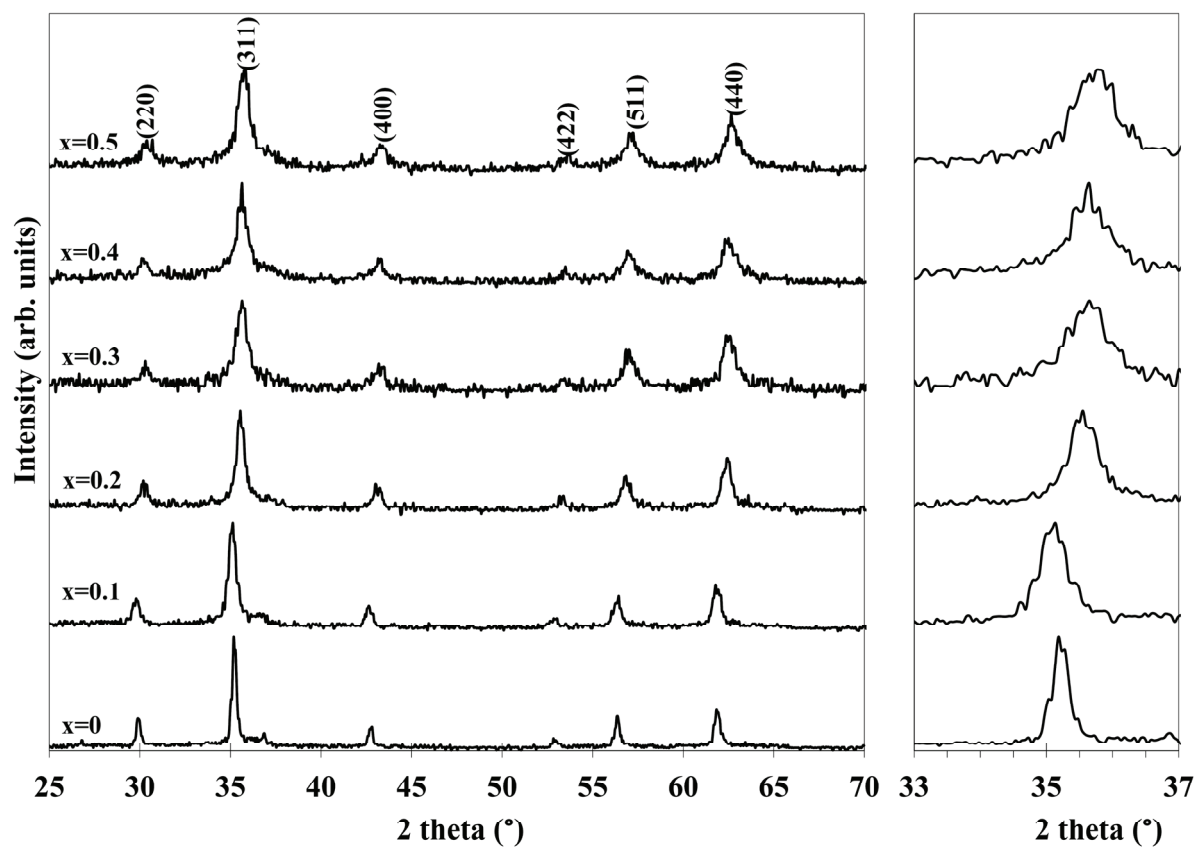
شکل ۱- (الف) الگوهای XRD فریت‌های نانوذرات \text{Mn}_{1-x}\text{Co}_x\text{Fe}_2\text{O}_4 و (ب) جابه جایی پیک پراشی (۳۱۱) بر حسب مقدار x
