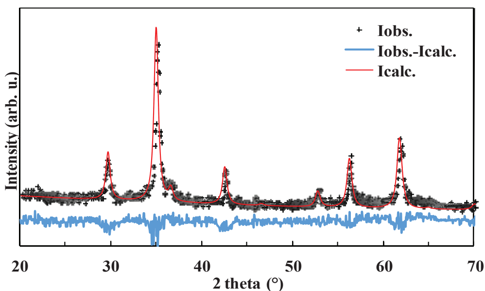
شکل ۲- الگوی XRD و نتایج رایتولد پودرهای هم‌رسوبی شده \text{Mn}_{0.9}\text{Co}_{0.1}\text{Fe}_2\text{O}_4
