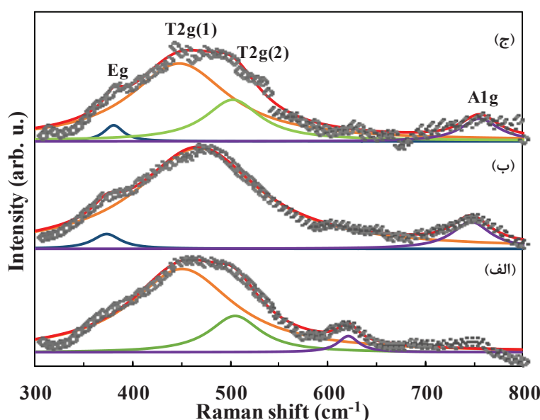
شکل ۳- طیف‌های رامان نانوذرات (الف) \text{MnFe}_2\text{O}_4 ، (ب) \text{Mn}_{0.8}\text{Co}_{0.2}\text{Fe}_2\text{O}_4 و (ج) \text{Mn}_{0.7}\text{Co}_{0.3}\text{Fe}_2\text{O}_4
