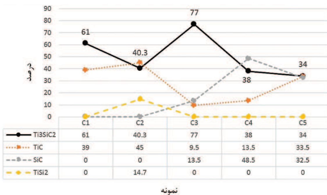
شکل ۲- نمودار تغییرات درصد فازهای نمونه‌های C1 تا C5.
