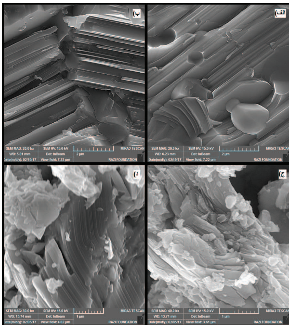
شکل ۶- تصاویر FE-SEM ساختار نانولایه‌ای مکس فاز \text{Ti}_3\text{SiC}_2 .
