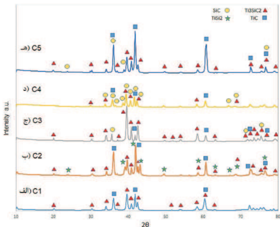
شکل ۱- الگوی پراش اشعه X نمونه‌هایی با پیش‌سازهای الف) TiC ، ب) TiC/Ti ، ج) 3TiC/0.3Si ، د) Ti/C (کربن اکتیو) و ه) Ti/C (گرافیت).
