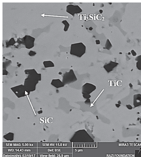
شکل ۳- تصویر الکترون برگشتی (FE-SEM) نمونه C3 که با ترکیب پیش‌ساز 3TiC/0.3Si، زمان آسیاب ۱۵ دقیقه، فشار پرس ۸۰ MPa و ۳ برابر مقدار استوکیومتری شمش Si سنتز شده است.
