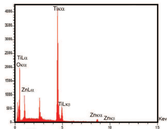
شکل ۳- تصویر EDX نانوکامپوزیت‌های هسته/پوسته ZnO/TiO_2
