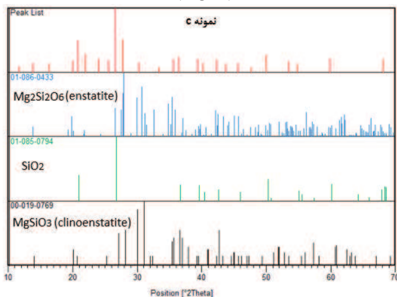
شکل ۳- (الف) طیف‌های پراش اشعه ایکس نمونه‌های انگوب (ب) نمودار تحلیل قله‌های پراش نمونه C (مثال)
