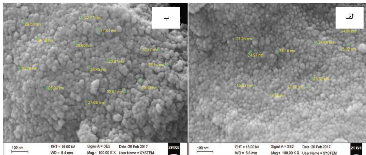
شکل ۲- تصاویر FESEM نانوذرات \text{TiO}_2 (الف) نمونه خالص و (ب) نمونه آلائیده شده با سرب
