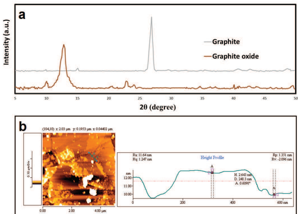
شکل ۳- طیف XRD و تصویر AFM نانوصفات گرافن اکساید
