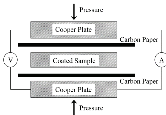
شکل ۱- شمایی از دستگاه طراحی شده برای اندازه‌گیری مقاومت تماسی.
