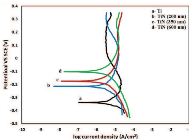
شکل ۶- نمودار نتایج تست پلاریزاسیون متغیر برای زیر لایه تیتانیومی، پوشش TiN با ضخامت ۲۰۰، ۳۵۰ و ۶۰۰ نانومتر.
