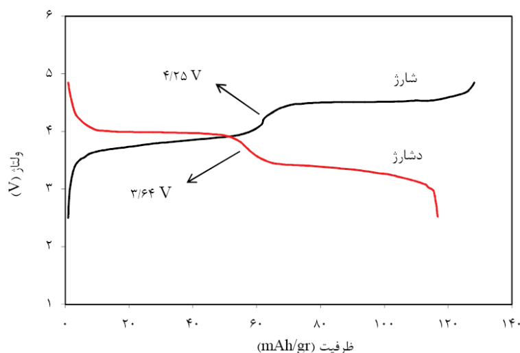
شکل ۷- منحنی های شارژ و تخلیه باتری کامل با کاند LMO و آند گرافیت با لایه محافظ LAGP در نرخ جریان ۰.۵ C.
