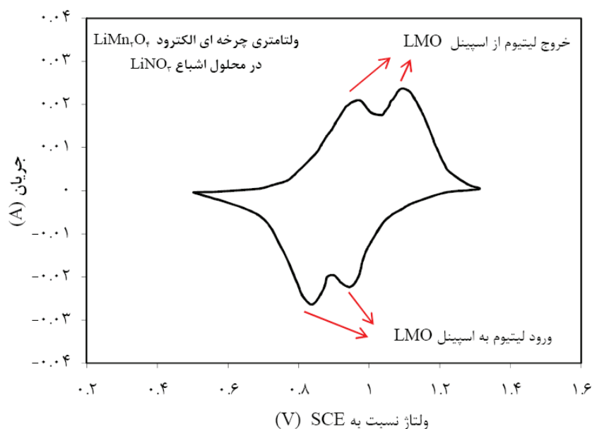
شکل ۶- تصویر ولتاموگرام چرخه‌ای مربوط به کاتد \text{LiMn}_2\text{O}_4 در محلول اشباع نیترات لیتیوم با نرخ روبش 1 mV/s
