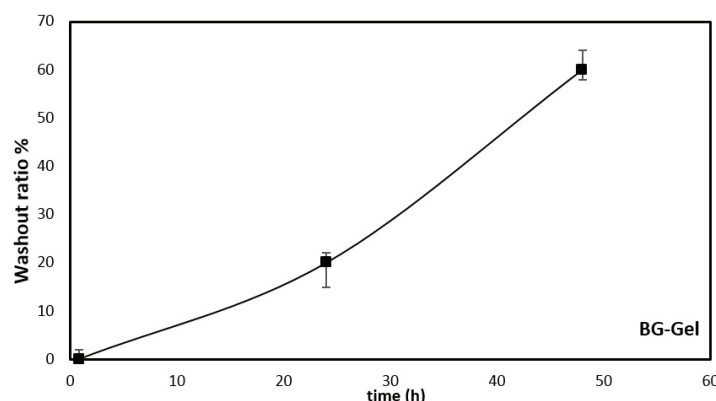
شکل ۹- منحنی آبشویی- زمان خمیر کامپوزیتی
