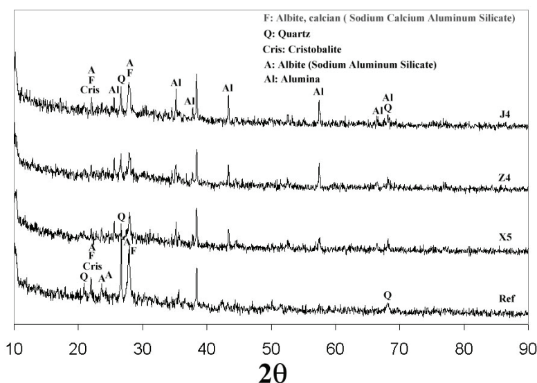
شکل ۷- الگوی پراش پرتو اشعه ایکس نمونه‌ها
