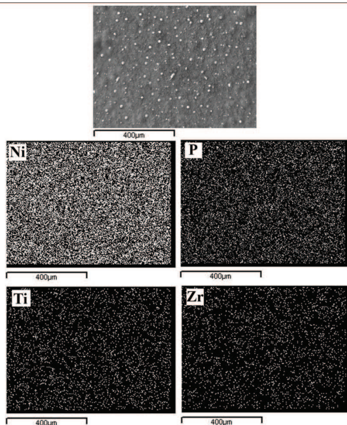
شکل ۴- تصویر SEM و آنالیز mapping از پوشش کامپوزیتی Ni-P-ZrO 2 -TiO 2
