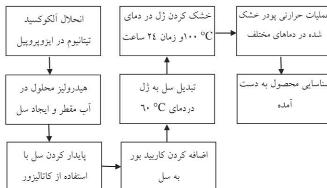
شکل ۱- فلوچارت مسیر بر پایه سل ژل در سنتز نانوذرات TiB_2
