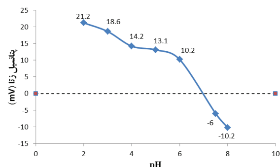
شکل ۴- اثر pH بر پتانسیل زتای سل حاوی ذرات پیش‌سازنده
