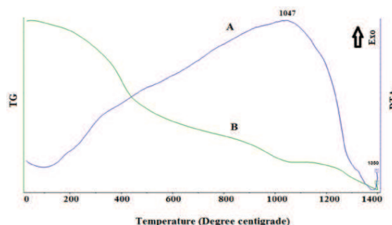
شکل ۶- منحنی‌های آنالیز حرارتی افتراقی و تغییرات وزنی نمونه در دماهای مختلف مربوط به ژل نهایی
