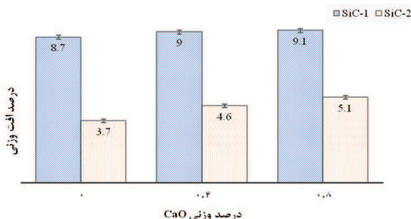
شکل ۴- درصد افت وزنی نمونه‌های سینتر شده از دو پودر SiC-1 و SiC-2 در مقادیر مختلف افزودنی \text{CaO} .
