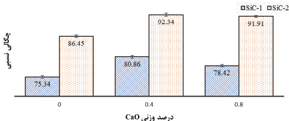
شکل ۳- تغییرات چگالی نسبی نمونه‌های سینتر شده از دو پودر SiC-1 و SiC-2 در مقادیر مختلف افزودنی \text{CaO} .
