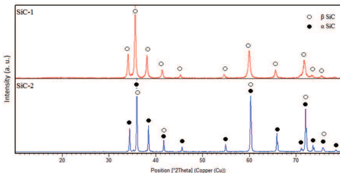
شکل ۱- الگوی پراش اشعه ایکس دو نوع پودر \text{SiC-1} و \text{SiC-2} .
