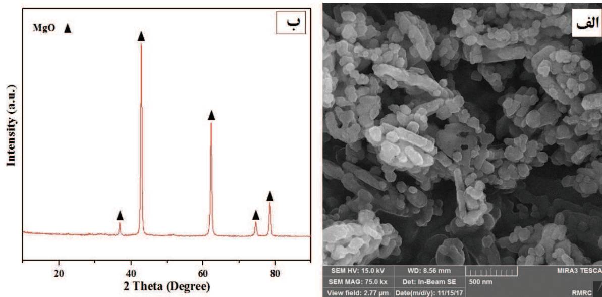
شکل ۱- الف) تصویر میکروسکوپ الکترونی روبشی و ب) الگوی پراش پرتو ایکس از نانوپودر منیزیای آسیاکاری شده به مدت ۱۵ ساعت در محیط اتانول و خشک شده در دمای 100^{\circ}\text{C} و سپس عبور داده شده از الک با مش ۲۳۰
