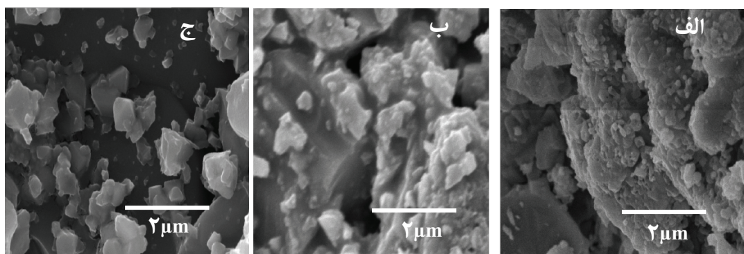
شکل ۳- تصاویر SEM پودرهای حاصل سنتز شده، الف) A_1 ب) A_2 ج) A_3
