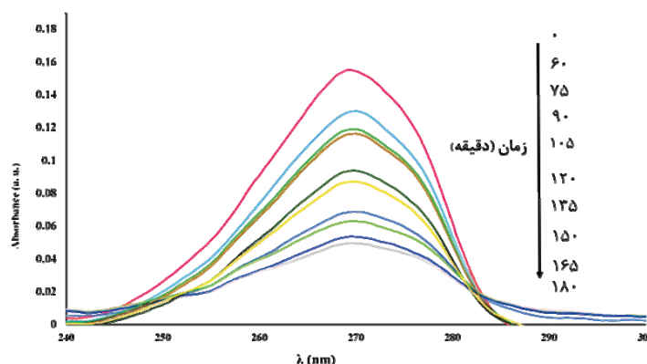
شکل ۴- کاهش پیک جذبی فنول با گذشت زمان توسط \text{Hap/Pd/Bi}_2\text{WO}_6 .
