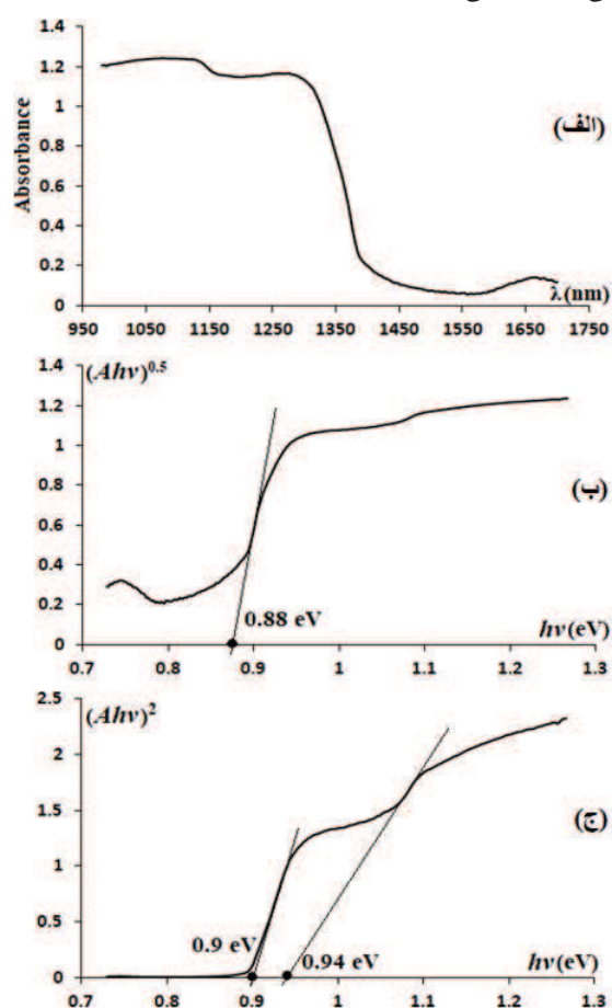
شکل ۶- (الف) طیف جذبی NIR از \text{Ag}_2\text{O}_2 سنتز شده؛
