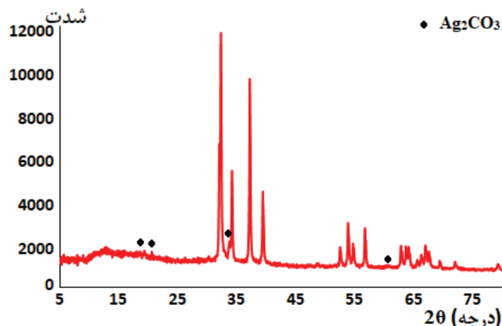
شکل ۲- الگوی XRD پودر سیاه به دست آمده از آزمایش.
