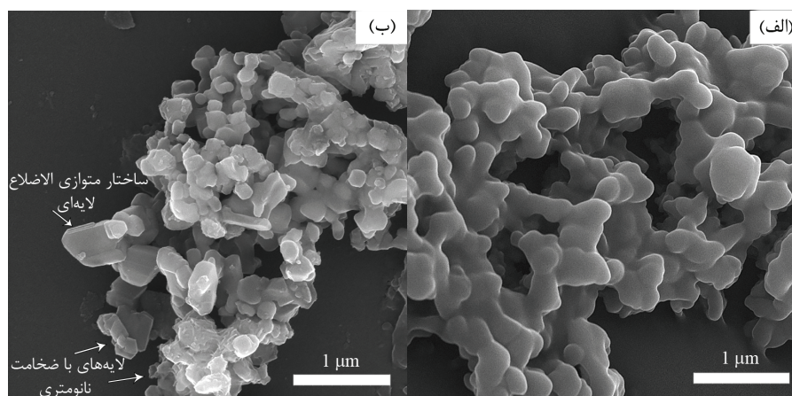
شکل ۵- تصویر SEM پس از اسید شویی از نمونه‌های آسیا (به مدت ۹ ساعت) و سپس سنتز شده در دستگاه جرقه پلاسما با قالب به قطر ۱/۵ (الف) و ۳ cm (ب) به منظور ایجاد درجای کامپوزیت کاربید بور-کاربید سیلیسیم به روش سنتز احتراقی حجمی.
