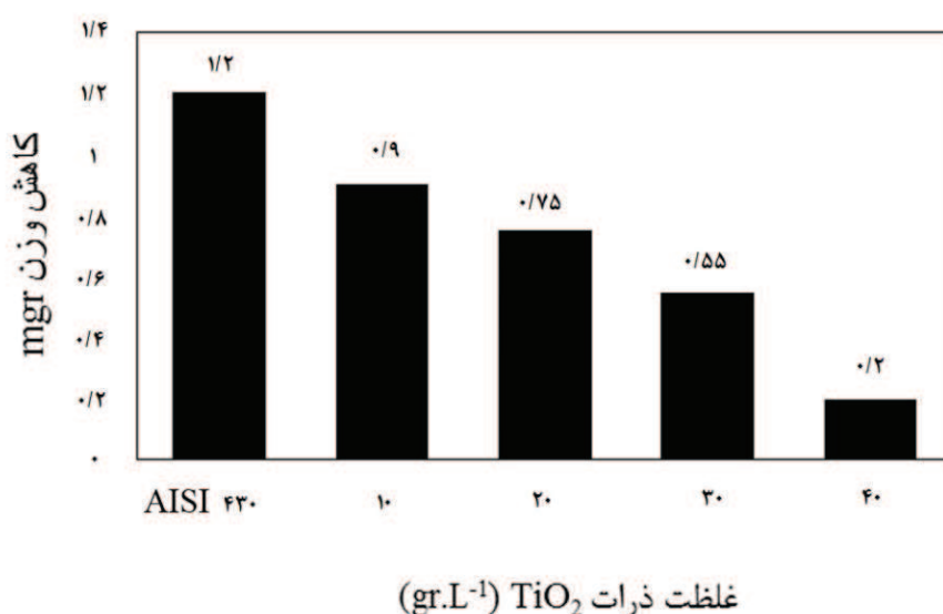
شکل ۷- تأثیر مقدار کاهش وزن نمونه ها را با تغییر غلظت ذرات \text{TiO}_2 در الکترولیت، تحت دانسیته جریان 15 \text{ mA.cm}^{-2} و \text{pH}=3/5 .
