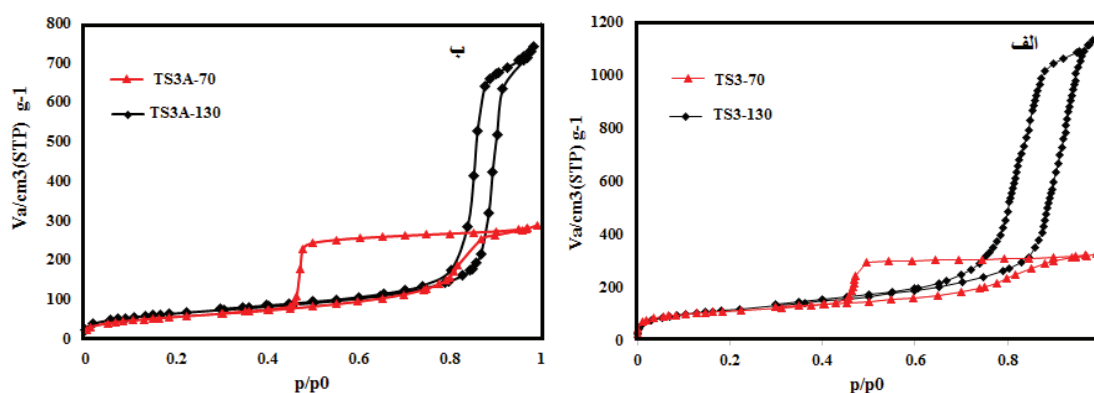
شکل ۳- ایزوترم جذب-واجذب (الف) نمونه‌های TS3-70، TS3-130، (ب) نمونه TS3A-70 و TS3A-130
