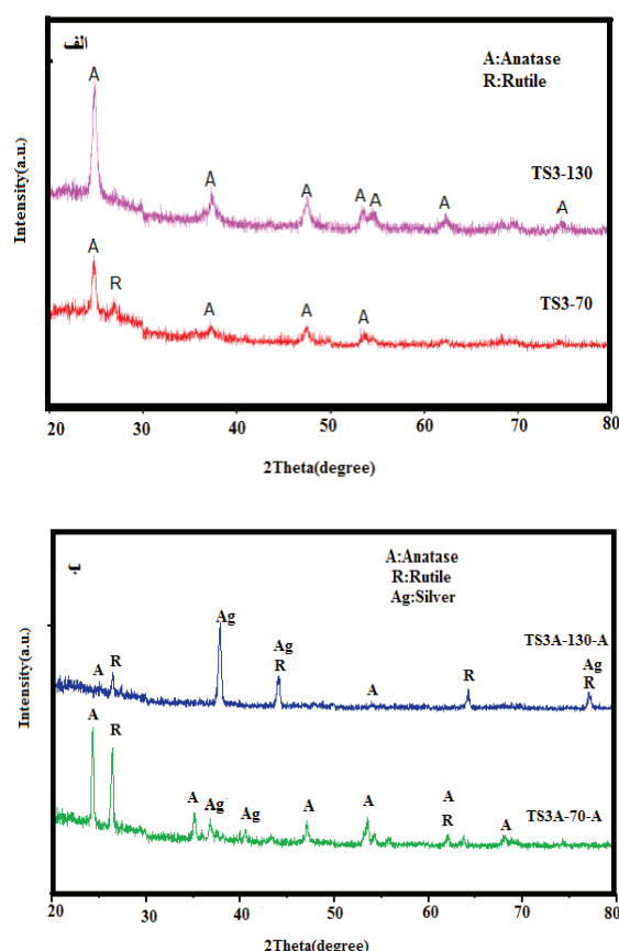
شکل ۱- الگوی پراش پرتو ایکس (الف) نانو کامپوزیت \text{TiO}_2\text{-SiO}_2 (ب) نانو کامپوزیت \text{SiO}_2\text{-TiO}_2 ۵٪ Ag
