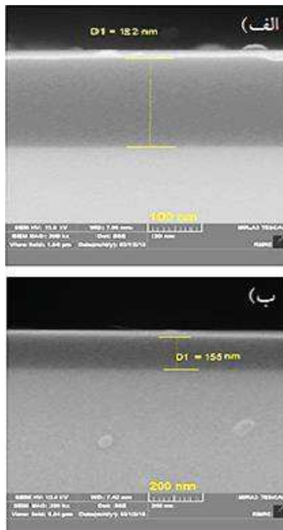
شکل ۹- تصاویر مقطعی FESEM از پوشش کربن شبه الماس ایجاد شده در ولتاژ بایاس (الف) ۱۰۰ V- و (ب) ۵۰ V-.
