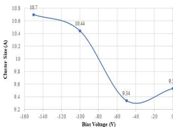
شکل ۷- اندازه خوشه‌های نانوغرافیتی پوشش کربن شبه‌الماس در ولتاژ بایاس 0\text{ V} ، 50\text{ V} ، 100\text{ V} و 150\text{ V} .
