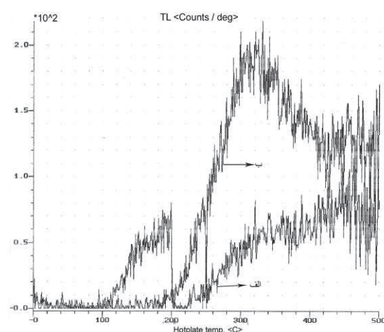
شکل ۴- نمودار ترمولومینسانس نمونه شماره ۱ (نگارندگان)
