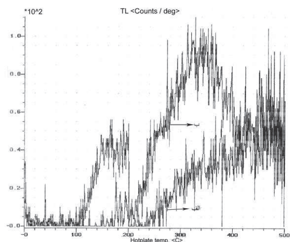
شکل ۵- نمودار ترمولومینسانس نمونه شماره ۲ (نگارندگان)
