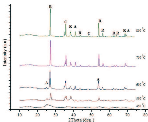
شکل ۹- الگوی پراش اشعه ایکس نمونه مزو متخلخل کامپوزیتی TiO 2 -CuO کلسینه شده در دماهای مختلف به مدت 1h (A: آنا تاز، R: روتایل، C: اکسید مس).
