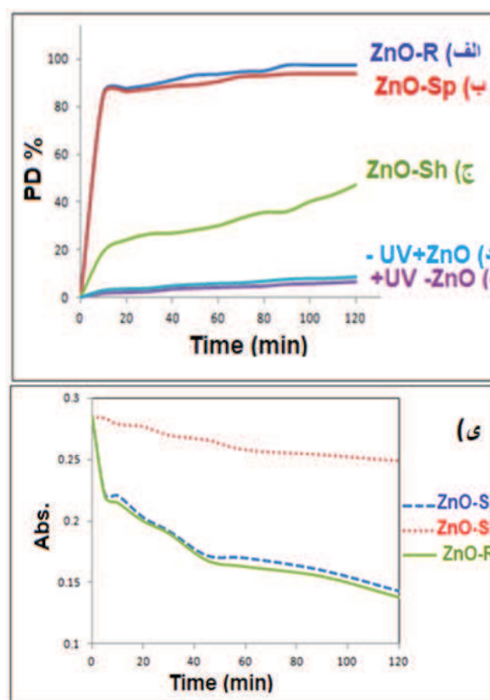
شکل ۶- نمودار تخریب نوری کنگورد بوسیله الف) ZnO-R در حضور اشعه UV ب) ZnO-Sp در حضور اشعه UV ج) ZnO-Sh در حضور اشعه UV د) ZnO-R در غیاب اشعه UV ه) اشعه UV در غیاب کاتالیست ی) نمودار جذب محلول PPM10 کنگورد توسط کاتالیست‌ها در غیاب اشعه UV
