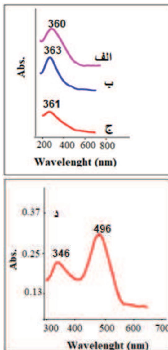
شکل ۳- طیف جذبی UV-Vis (الف ZnO-R، ب ZnO-Sp، ج ZnO-Sh) طیف جذبی کنگورد.
